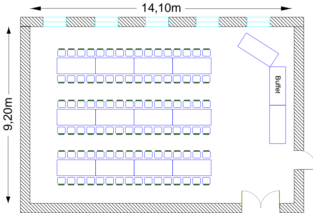
Tischreihen, Buffet Bestuhlung für 96 Personen
