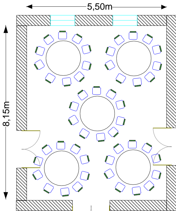
Reiterzimmer im 1. Obergeschoß
