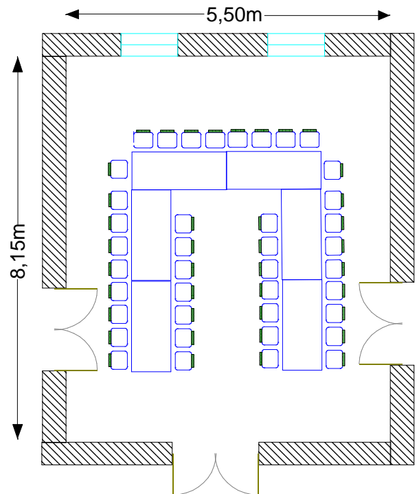
U-Form Bestuhlung für 40 Personen
